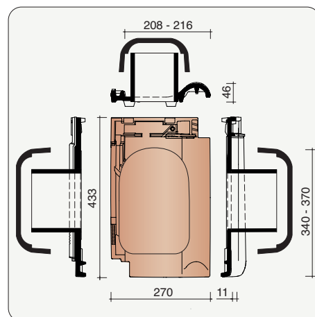
NTRA8728 Kit kokerpan + kapje Ø 125 mm + aansluitingsmodule + reductorstuk
