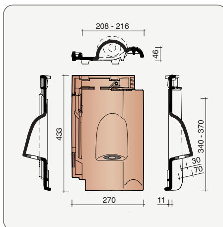
NTRA8958 Kabeldoorvoerpan Ø 70/30 mm
