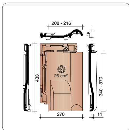
NTRA8640 Ventilatiepan/haakdoorvoerpan met rooster in kunststof 26 cm²
