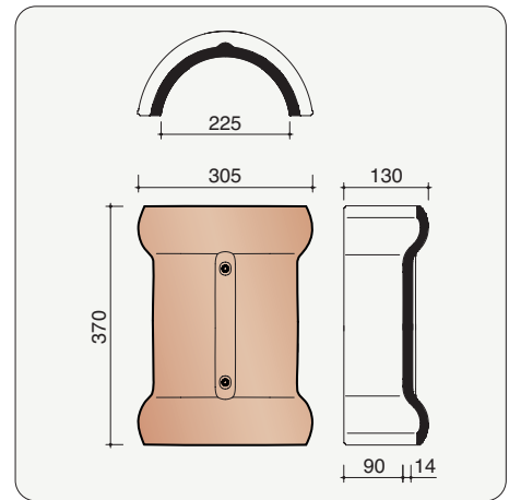
N0001250 Halfronde vorst Vario met dubbele wel - 225 mm
