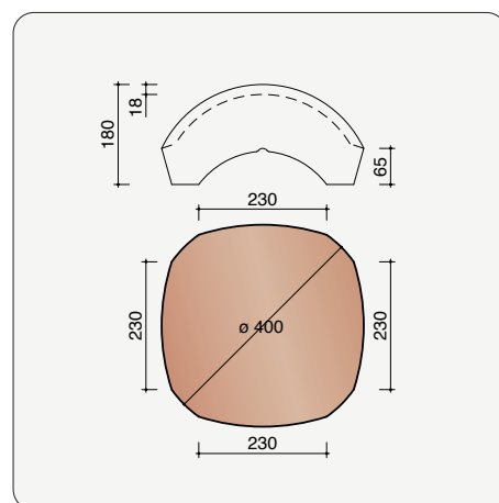
N0005540 Vorstenhoed als noordboom tussen 4 vorsten 1200
