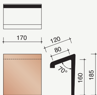
P3018510 5,9 stuks/lm Haakvorst 70°
