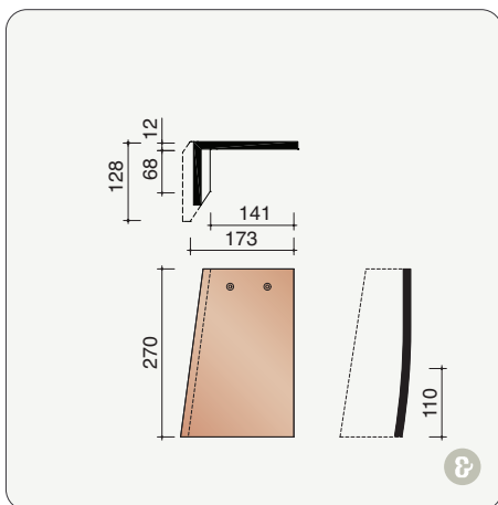
P3017080 4,5 stuks/lm Linker gevelpan
