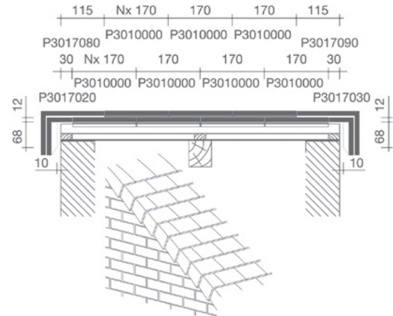
12 * Dwarsdoorsnede dak ter hoogte van gevelpan Frans systeem
