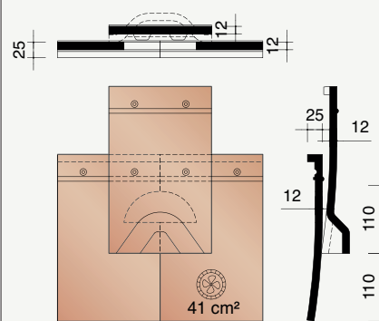
P3018611 Kit ventilatiepan met rooster - 41 cm 2
