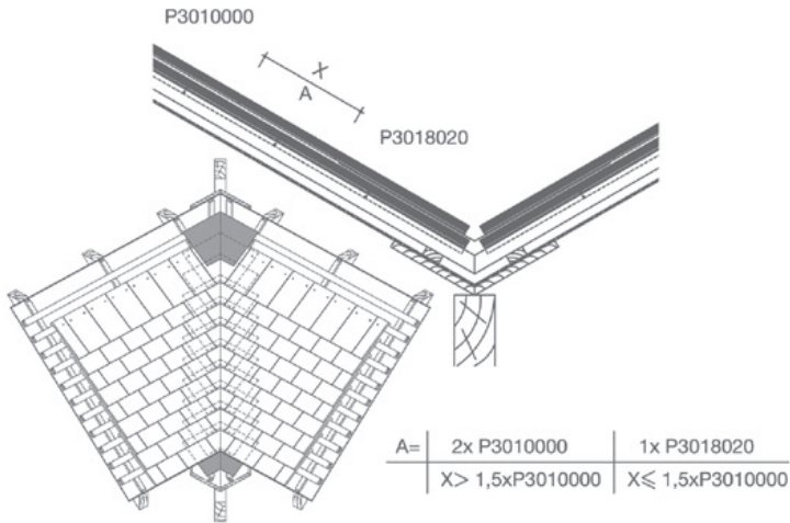
8 Doorsnede dak ter hoogte van kielgoot met ingewerkte loodvanger Koraflex (plus)
