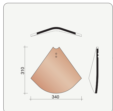
P3013470 9,1 stuks/lm Ingewerkte noordboom 35°
