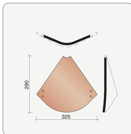
P3013180 9,1 stuks/lm Ingewerkte slaper (kielgoot) bij dakhelling van 45°
