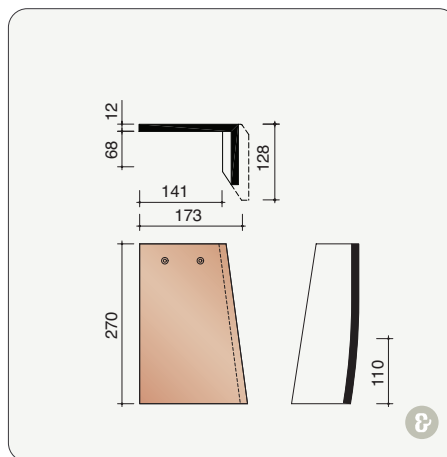
P3017090 4,5 stuks/lm Rechter gevelpan
