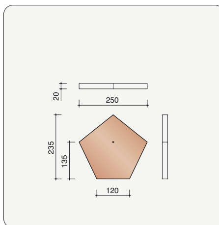
P0000510 Beginkopplaat voor spitsvorst
