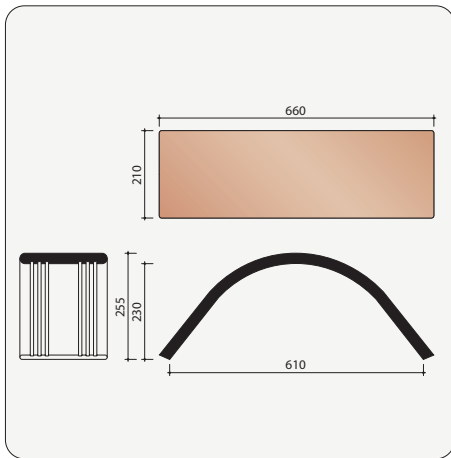
P0000010 4,5 stuks/lm Strovorst (Natuurrood of Bruin)
