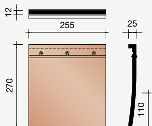
P3018020 Anderhalve pan
