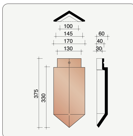
P0003410 Hoekige beginnoordboom
