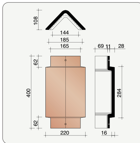
P0001830 Hoekige beginvorst zonder kopplaat
