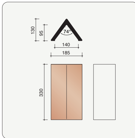
P0000400 3 stuks/lm Lessenaarsvorst
