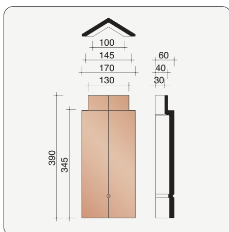
P0003400 2,9 stuks/lm Hoekige noordboom
