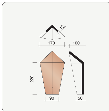
P0003710 Kleine hoekige beginnoordboom
