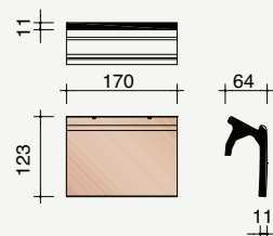
P3018200 5,9 stuks/lm Knikpan
