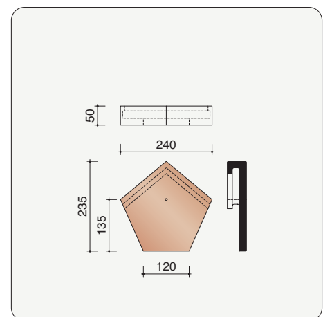
P0000540 Eindkopplaat voor spitsvorst
