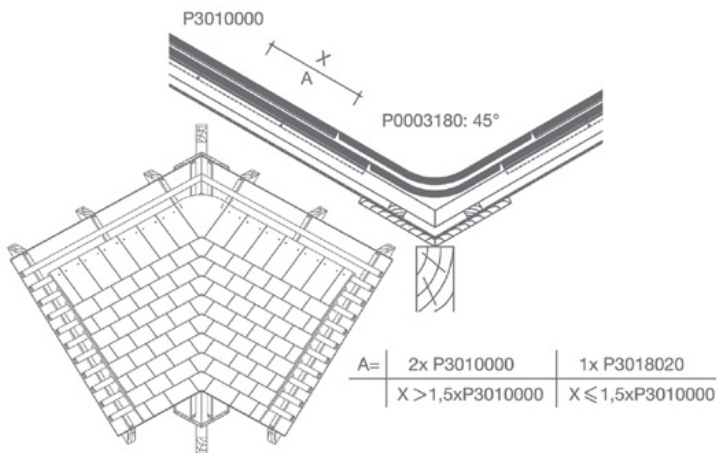
10 Doorsnede dak ter hoogte van kielgoot in metaal
