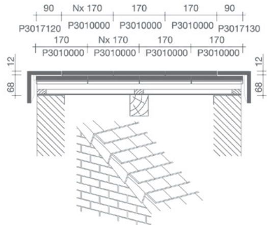
13 * 3d tekening gevelbekleding met doorsnede
