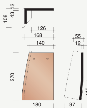
P3018800 4,5 stuks/lm Linker hoekstuk (gevelbekleding)
