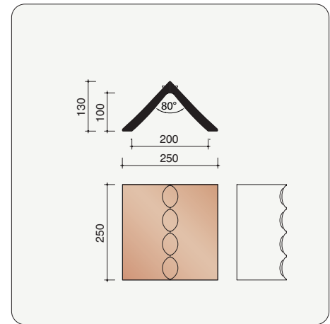
P0000200 4 stuks/lm Speciale vorst met "Duimslag"
