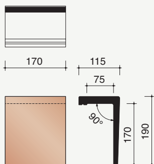
P3018520 5,9 stuks/lm Haakvorst 90°
