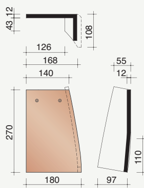
P3018810 4,5 stuks/lm Rechter hoekstuk (gevelbekleding)
