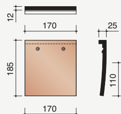
P3018110 5,9 stuks/lm Korte pan
