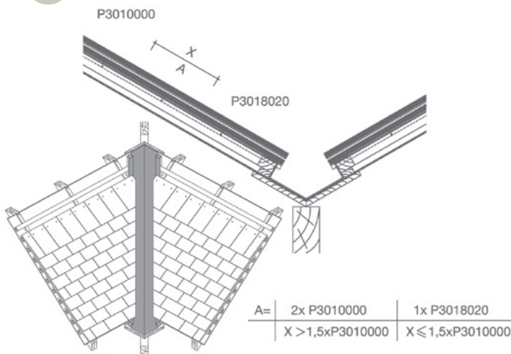
10 Doorsnede dak ter hoogte van kielgoot in metaal
