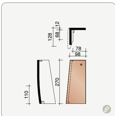
P3017120 4,5 stuks/lm Speciale linker halve gevelpan
