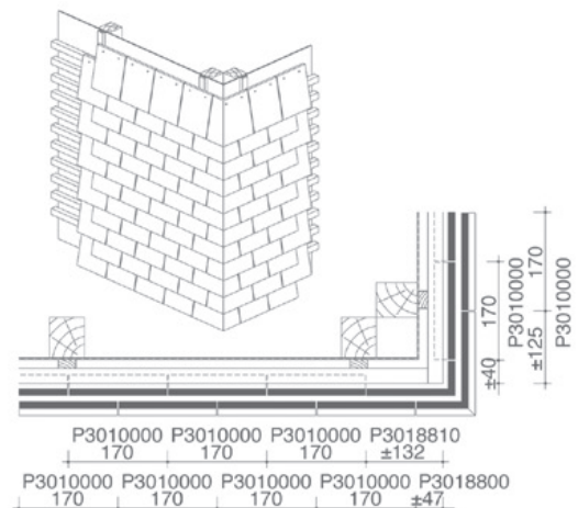
13 * 3d tekening gevelbekleding met doorsnede
