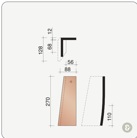
P3017020 4,5 stuks/lm Linker halve gevelpan
