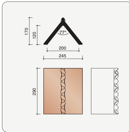
P0000100 3,4 stuks/lm Speciale vorst met "Duimslag" - oud model
