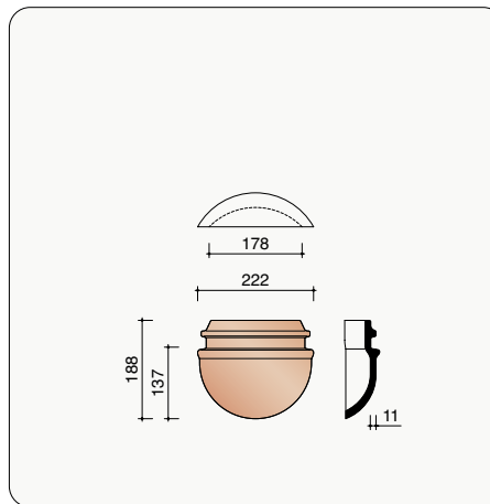
P0003110 Halfronde beginnoordboom - 190 mm
