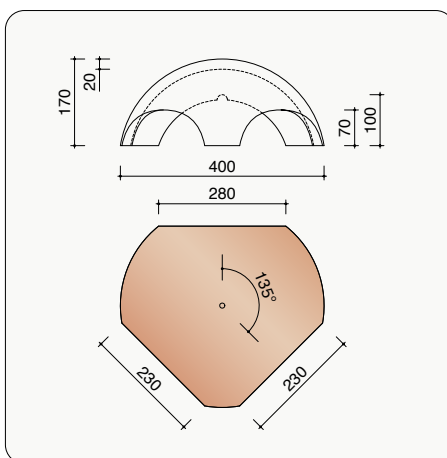
P0005740 Vorstenhoed tussen 1 vorst 1200 en 2 noordbomen 3100
