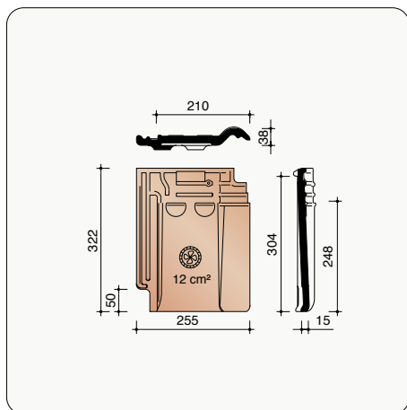
P9938610 Ventilatiepan/haakdoorvoerpan - 12 cm²
