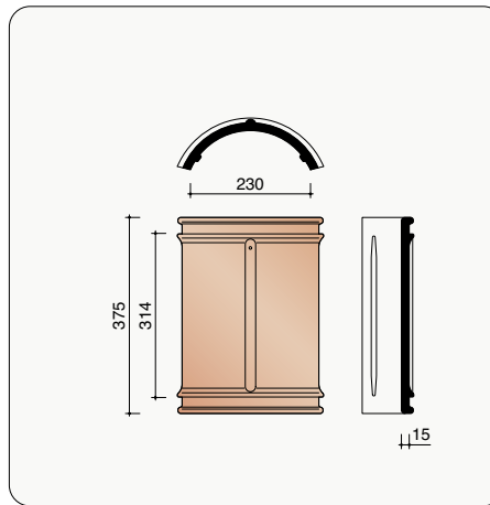
P0001230 Halfronde beginvorst/beginnoordboom - 230 mm
