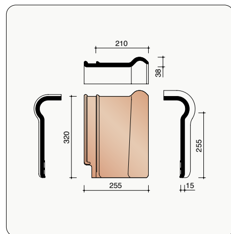
P9938500 4,8 stuks/lm Haakvorst
