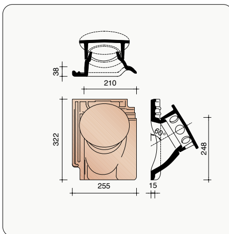
P9938741 Kit kokerpan Ø 100 mm + kapje - 95 cm² + aansluitingsmodule
