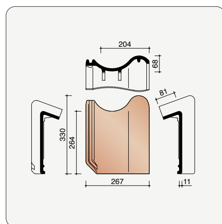
JOVH8500 4,9 stuks/lm Haakvorst
