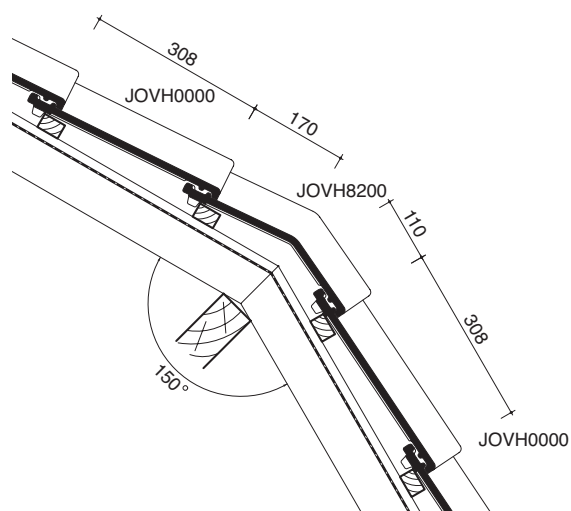
6 Lengtedoorsnede dak ter hoogte van knikpan
