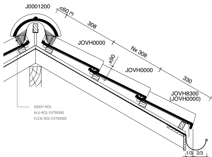
1 Lengtedoorsnede dak ter hoogte van vorst
