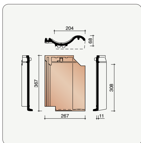
JOVH8300 4,9 stuks/lm Pan met gebogen board
