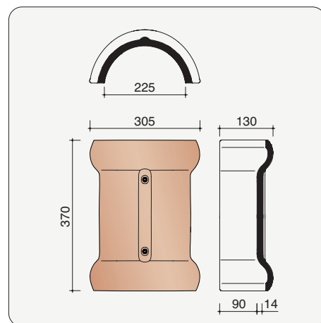
J0001250 Halfronde vorst Vario met dubbele wel - 225 mm
