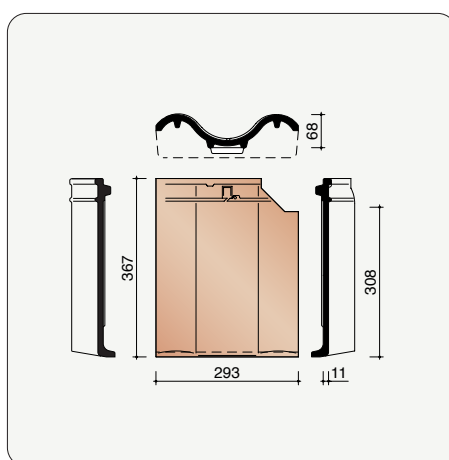
JOVH8350 Pan met gebogen board en dubbele wel
