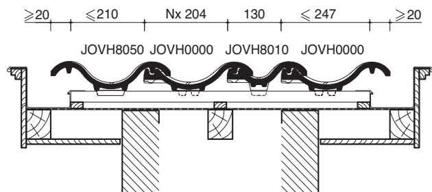
3 Dwarsdoorsnede dak ter hoogte van pan met dubbele wel
