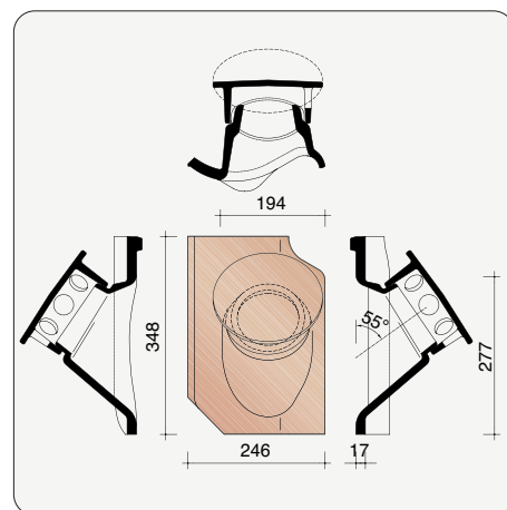
P4518741 Kit koperpan Ø 100 mm + kapje - 95 cm² + aansluitingsmodule
