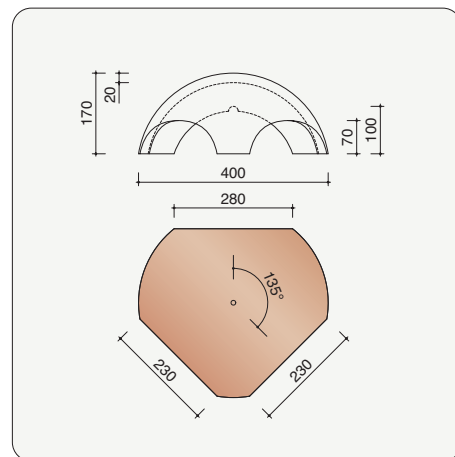
P0005740 Vorstenhoed tussen 1 vorst 1200 en 2 noordbomen 3100
