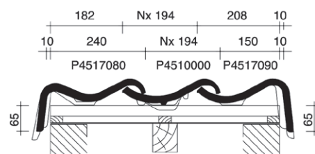
7 Dwarsdoorsnede dak ter hoogte van gevelpannen
