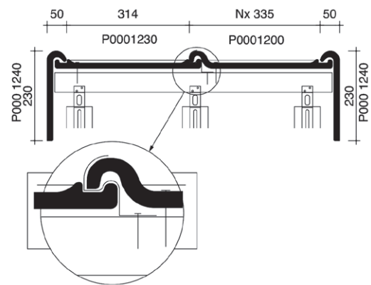
5 Dwarsdoorsnede dak ter hoogte van vorst zonder sluiting 1400 - Quick-Fix Extreme
