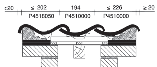
6 Dwarsdoorsnede dak met pan met dubbele wel
