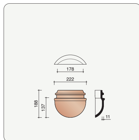
P0003110 Halfronde beginnoordboom - 190 mm
