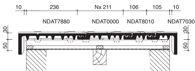
3 Lengtedoorsnede dak ter hoogte van haakvorst
