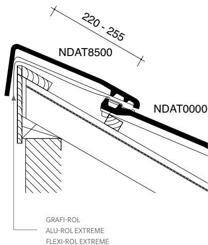
3 Lengtedoorsnede dak ter hoogte van haakvorst
