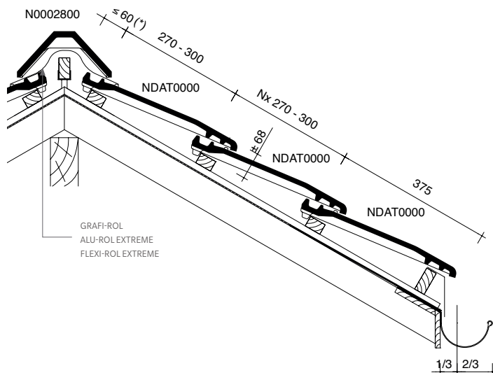
2 Dwarsdoorsnede dak ter hoogte van anderhalve linker en halve rechter gevelpan
