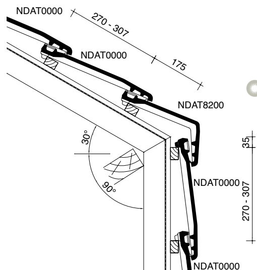
6 Lengtedoorsnede dak ter hoogte van knikpan
