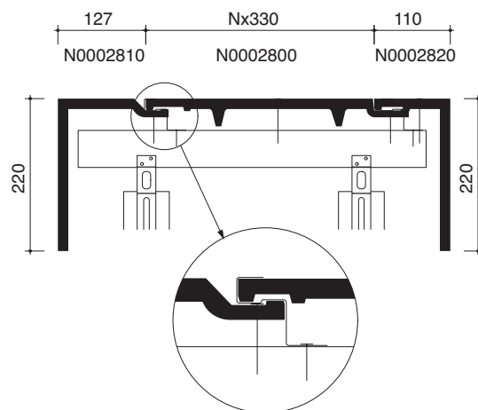
4 Dwarsdoorsnede dak ter hoogte van hoekige vorst 2800
