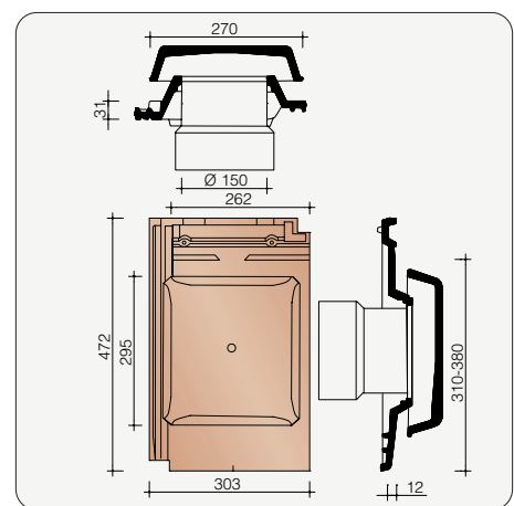
MACT8729 Kit kokerpan Ø 150 mm + kapje + aansluitingsmodule
