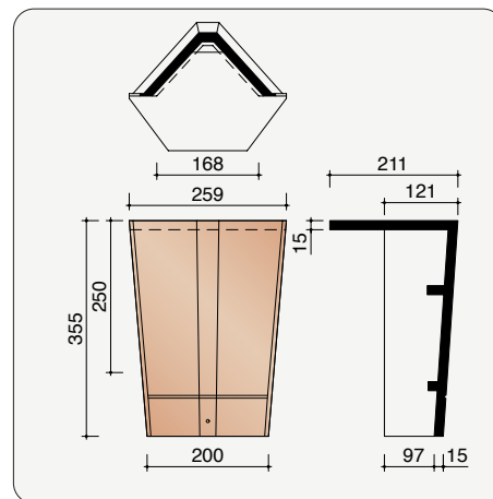
M0001910 Hoekige beginvorst Vauban
