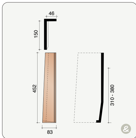
MACT7060 2,6 stuks/lm Linker gevelplaat
