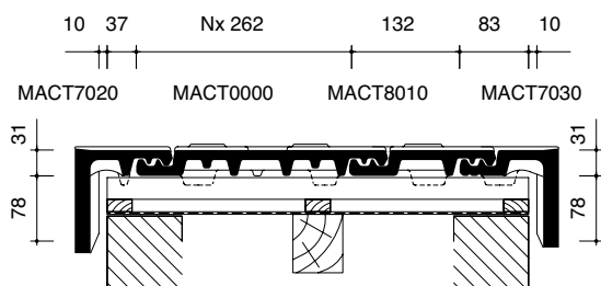
3 Dwarsdoorsnede dak ter hoogte van halve gevelpannen
