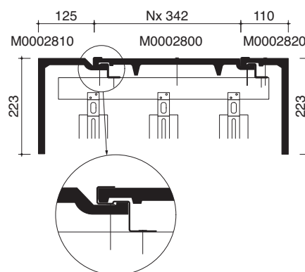
6 Dwarsdoorsnede dak ter hoogte van pan zonder zijsluiting
