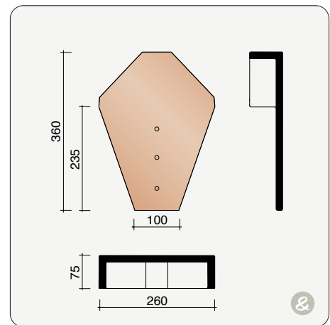
MACT2840 Hoekige kopplaat Actua 10
