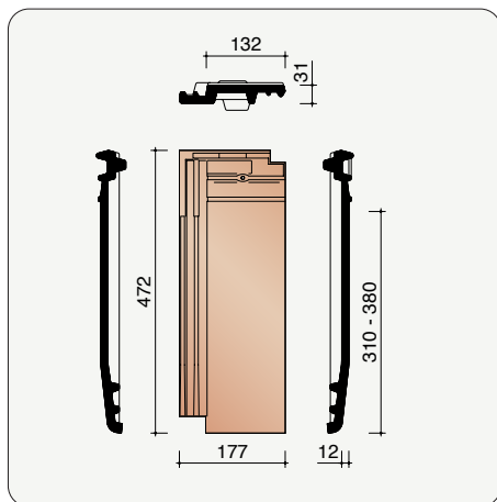
MACT8010 1,3 stuks/lm Halve pan
