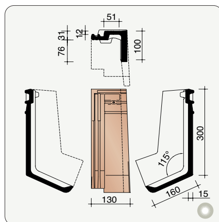
MACT7230 Rechter halve gevelknikpan op maat (verlijmd)
