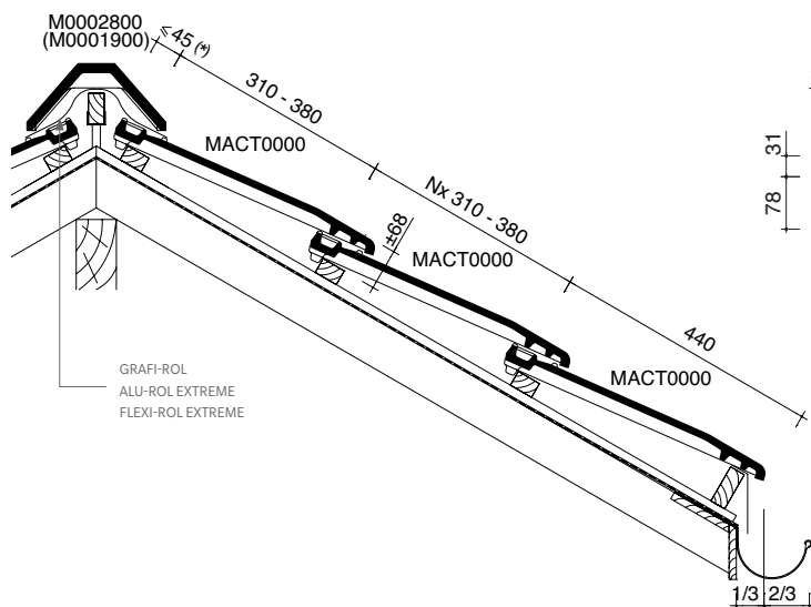
2 Dwarsdoorsnede dak ter hoogte van hoekige vorst Vauban
