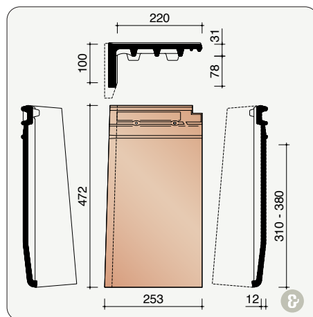
MACT7080 1,3 stuks/lm Linker gevelpan
