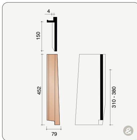
MACT7070 2,6 stuks/lm Rechter gevelplaat
