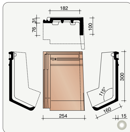
MACT7290 Rechter gevelknikpan op maat (verlijmd)
