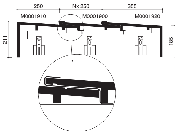
3 Dwarsdoorsnede dak ter hoogte van halve gevelpannen
