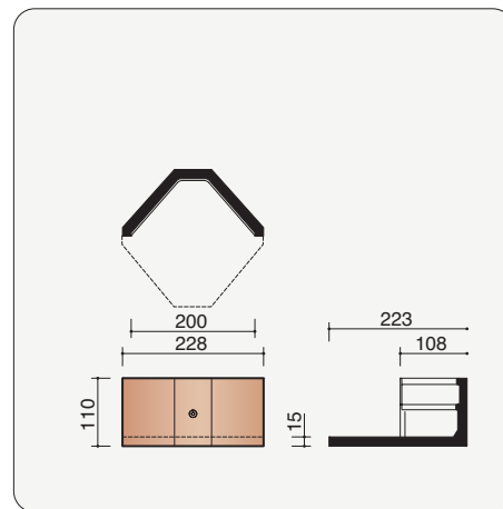
M0002820 Hoekige eindvorst Actua 10
