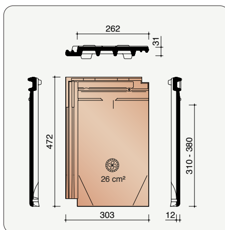
MACT8640 Ventilatiepan met rooster in kunststof - 26 cm 2
