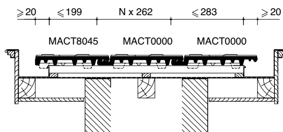
6 Dwarsdoorsnede dak ter hoogte van pan zonder zijsluiting
